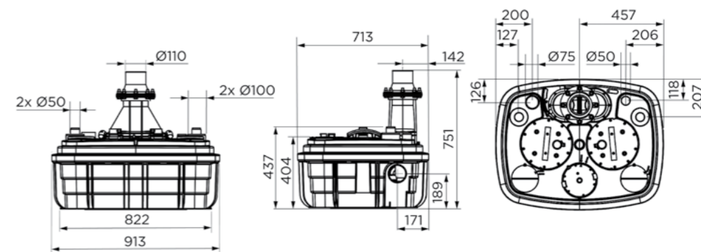
Размеры (мм)
